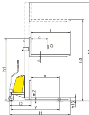
CDD10B - III / CDD15B - III Adjustable forks
