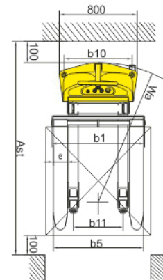
CDD10B - III / CDD15B - III Adjustable forks
